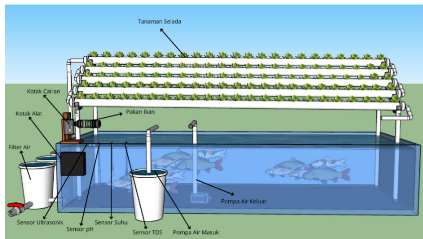
Gambar IV. 2 Tampak Depan Desain Sistem
