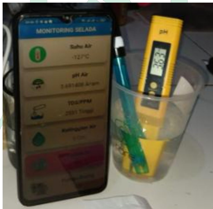
Lampiran 5. Pengujian Akurasi Sensor pH dengan bubuk pH 4.01
