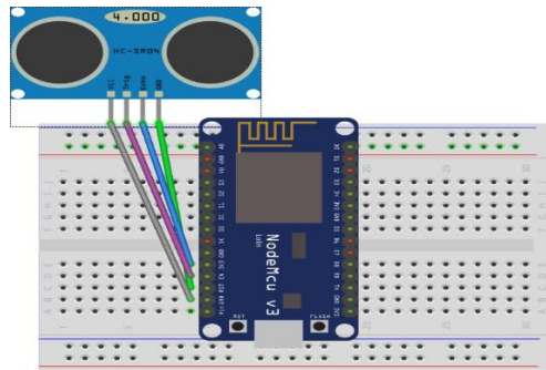
Gambar IV. 7 Perancangan Perangkat Keras Sensor Ultrasonik
