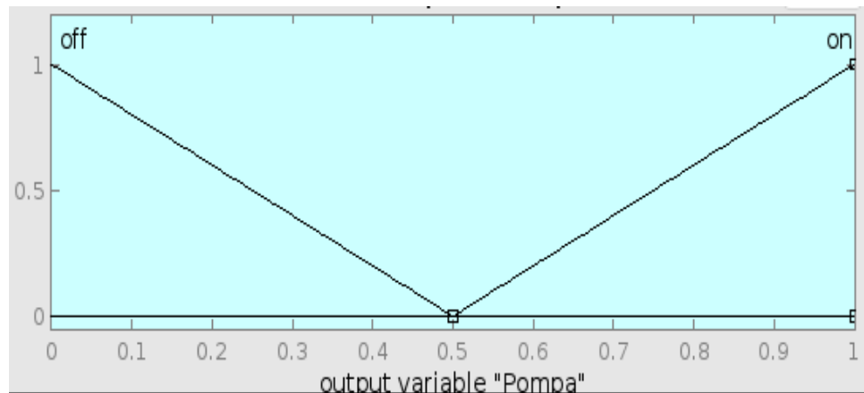
Gambar V. 10 Fungsi Keanggotaan Pompa
