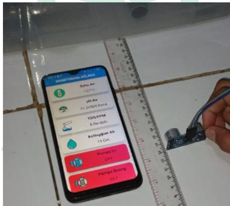
Lampiran 9. Pengujian sensor ultrasonic dengan mistar (15cm)
