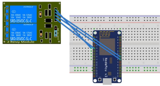
Gambar IV. 8 Perancangan Perangkat Keras Relay
