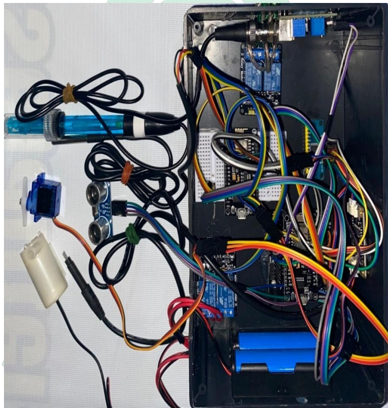
Gambar V. 1 Perancangan Perangkat Keras Keseluruhan
