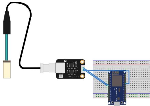
Gambar IV. 5 Perancangan Perangkat Keras Sensor pH
