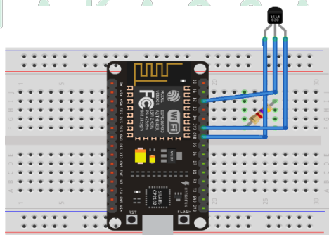
Gambar IV. 4 Perancangan Perangkat Keras Sensor Suhu DS18B20
