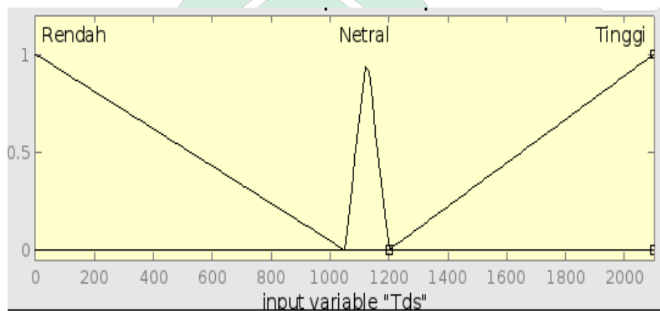
Gambar V. 9 Fungsi Keanggotaan TDS
