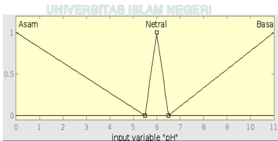
Gambar V. 8 Fungsi Keanggotaan pH
