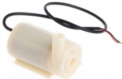
Gambar II. 10 Mini Pump Motor DC ( Sumber : www.digiwarestore.com )
